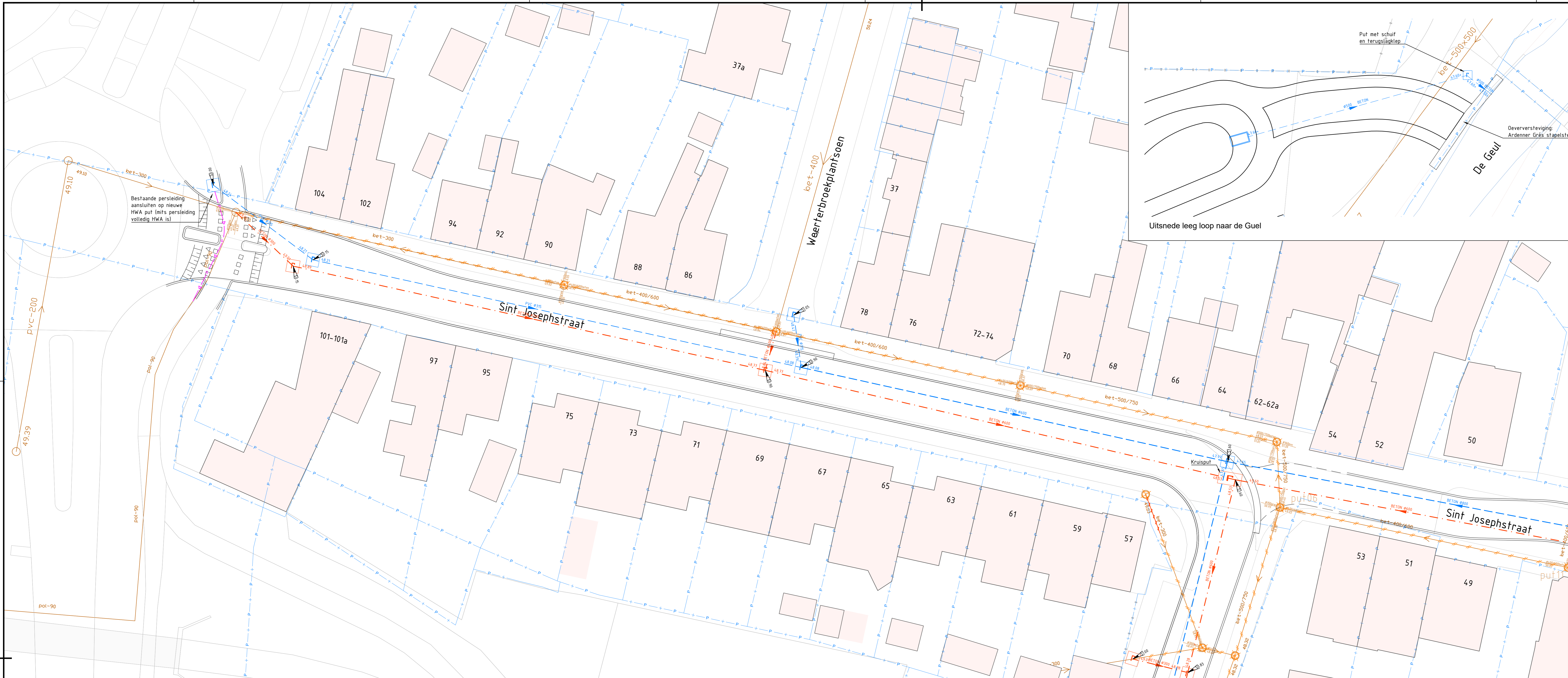
Uitsnede uitstroombuffer
