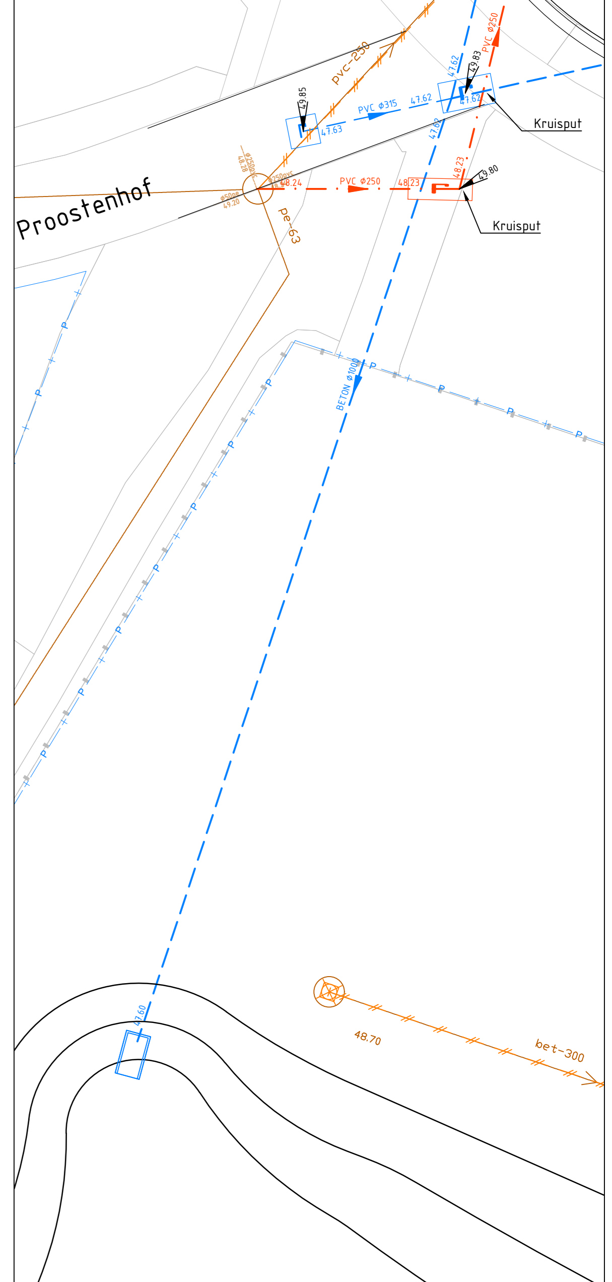
Uitsnede uitstroombuffer
